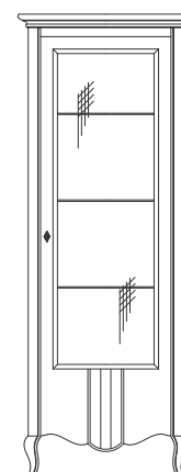
Cristalier 1 usa dreapta 1 Door glass cabinet - right Витрина 1 дверь - правая mm. 790 x 480 x H.2045
