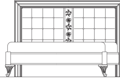
Pat dublu 1600 Double bed 1600 Двуспальная кровати 1600 mm. 1770 x 2180 x H.410/1250
