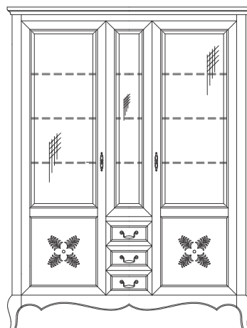
Cristalier 3 usi 3 Doors glass cabinet Витрина 3 двери mm. 1590 x 480 x H.2100
