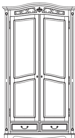
Dulap 2 usi 2 Doors wardrobe Шкаф 2 двери mm. 1240 x 670 x H.2270
