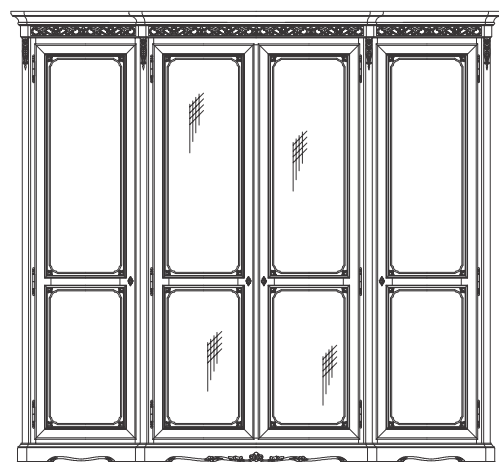
Dulap 4 usi 4 Doors wardrobe Шкаф 4 двери mm. 2410 x 650 x H.2240
