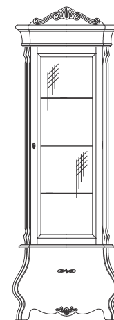
Cristalier 1 usa dreapta 1 Door glass cabinet - right Витрина 1 дверь - правая mm. 760 x 430 x H.2180
