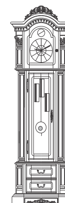
Carcasa ceas Clock case Каркас часы mm. 680 x 365 x H.2220
