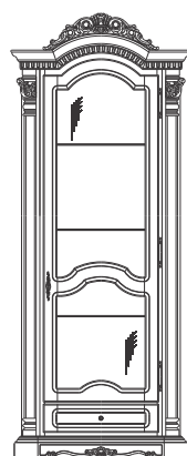
Cristalier 1 usa dreapta 1 Door glass cabinet – right Витрина 1 дверь - правая mm. 900 x 445 x H.2200
